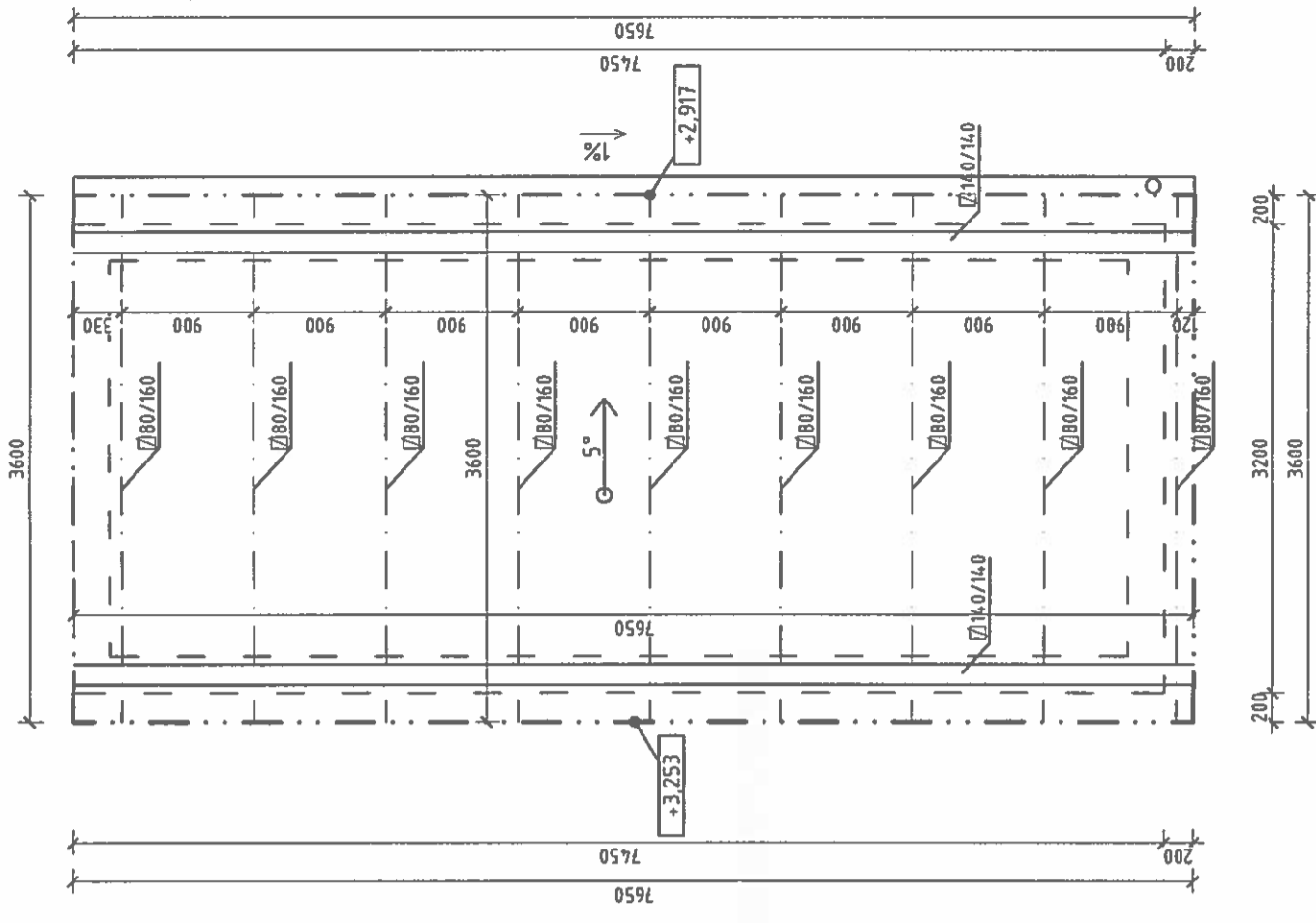
STRECHA M 1:50
