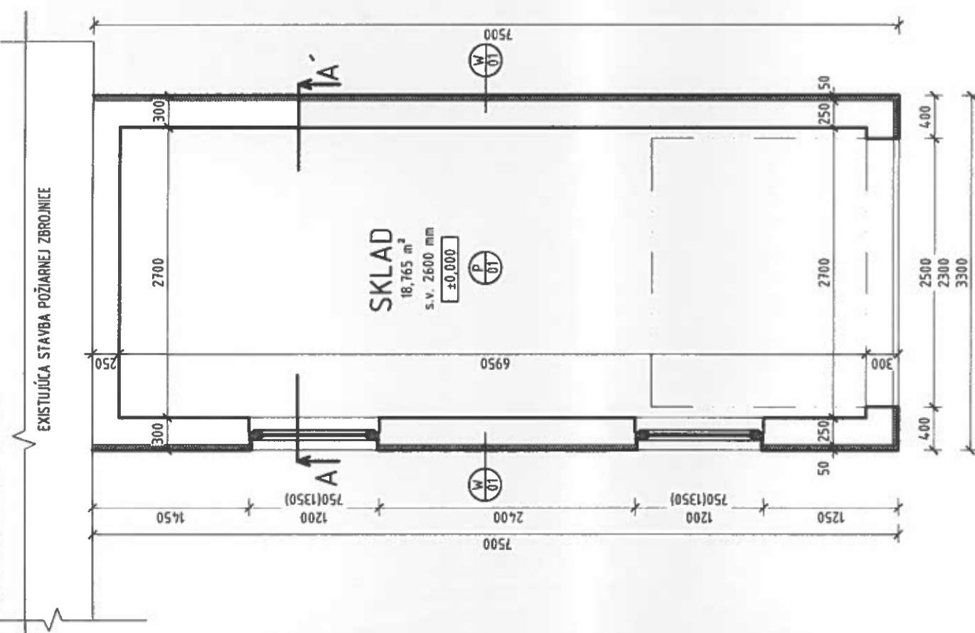
PŮDORYS 1.NP M 1:50
