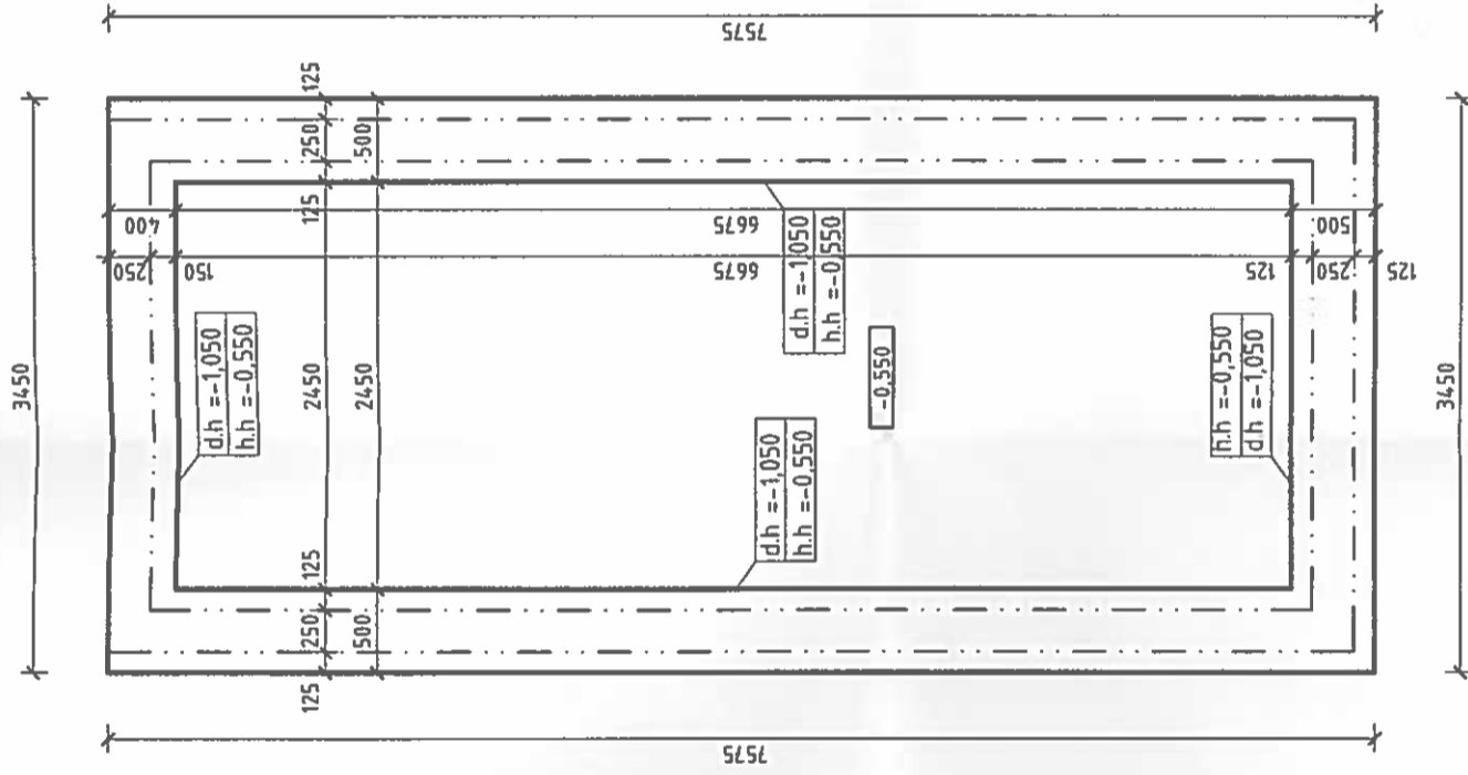
PŮDORYS ZÁKLADOV M 1:50
