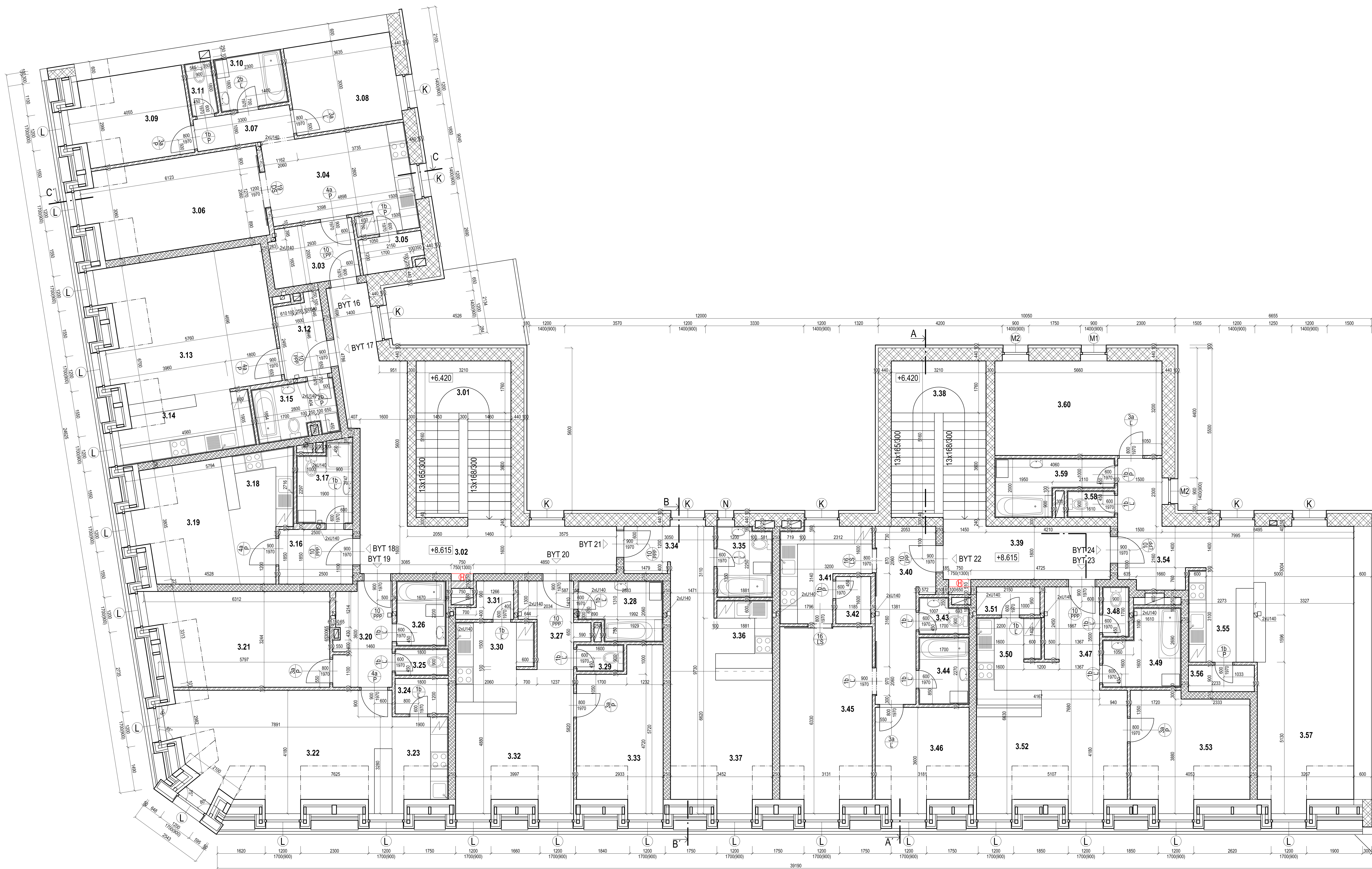
PÓDORYS PODKROVIA NAVRHOVANÝ STAV M 1:50
