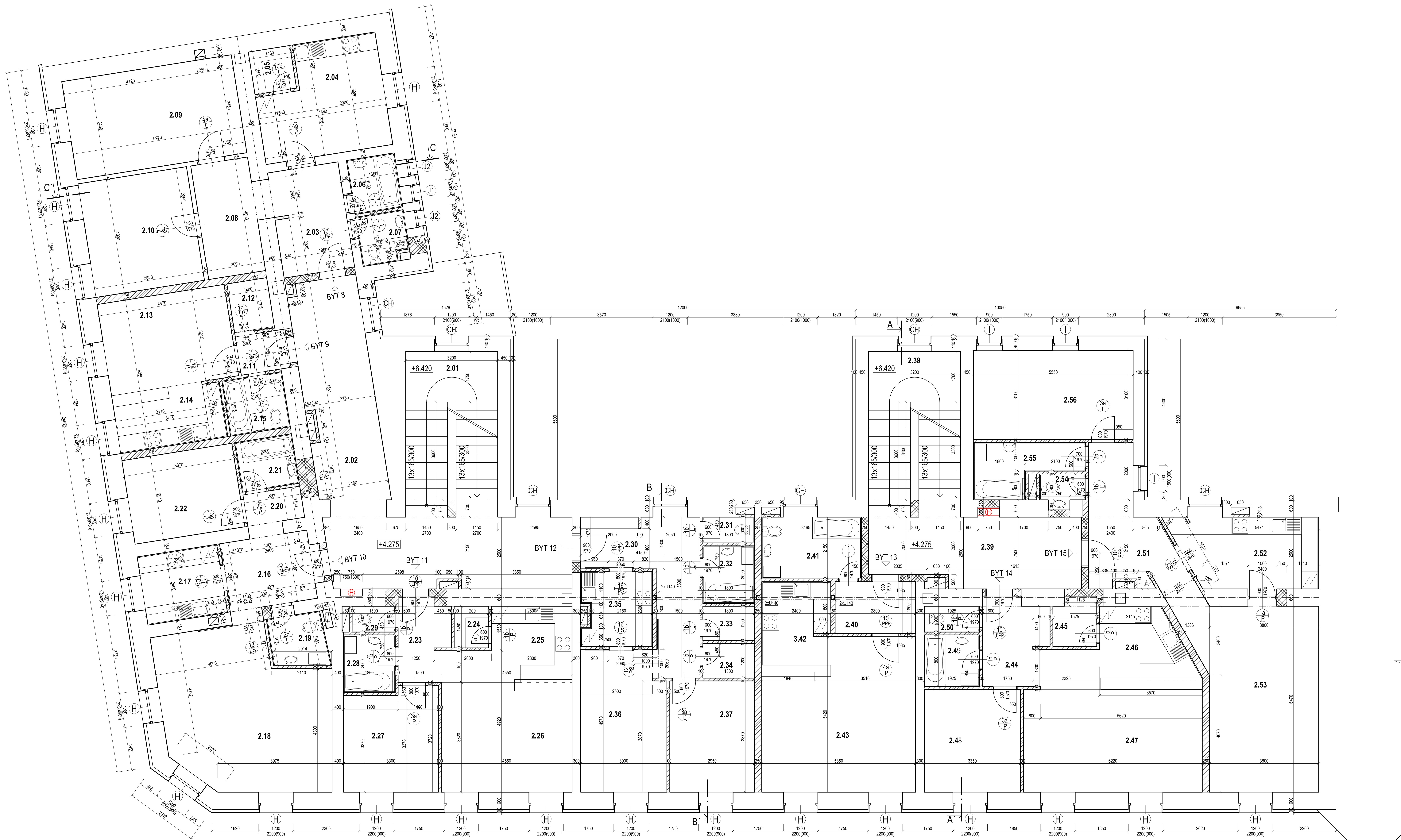
PÓDORYS 2.N.P. NAVRHOVANÝ STAV M 1:50
