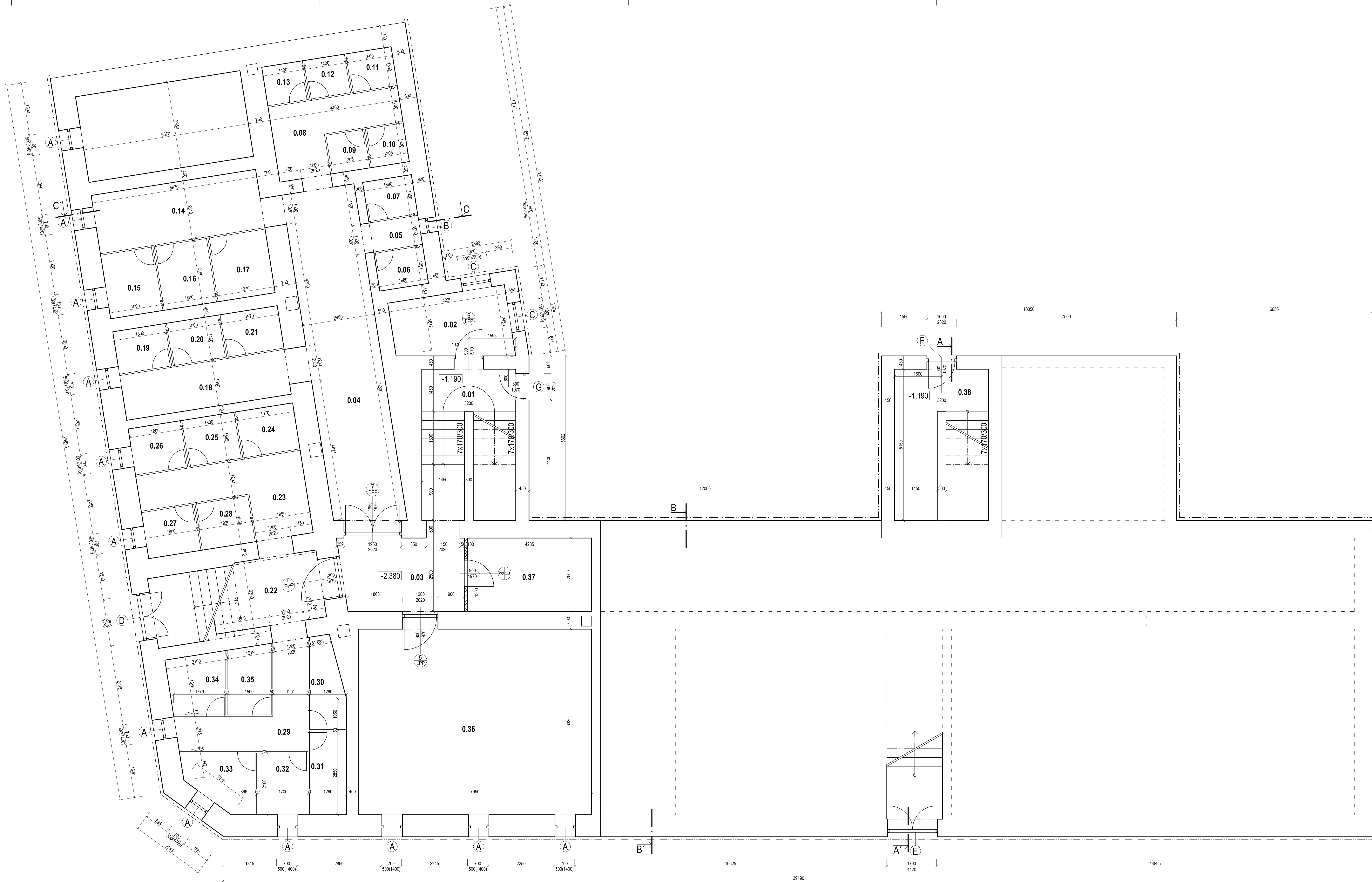
PÓDORYS 1.P.P. NAVRHOVANÝ STAV M 1:50
