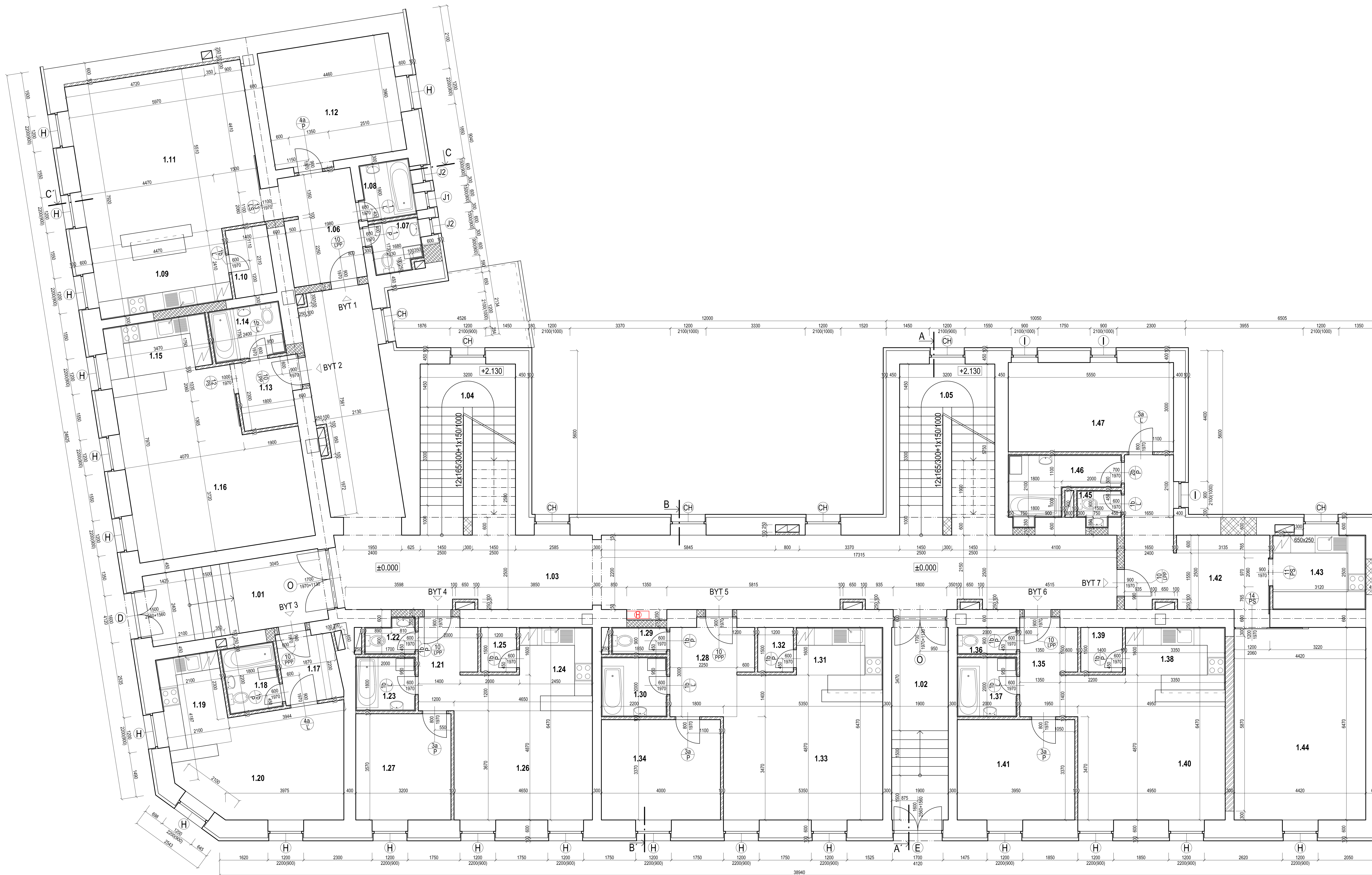
PÓDORYS 1.N.P. NAVRHOVANÝ STAV M 1:50
